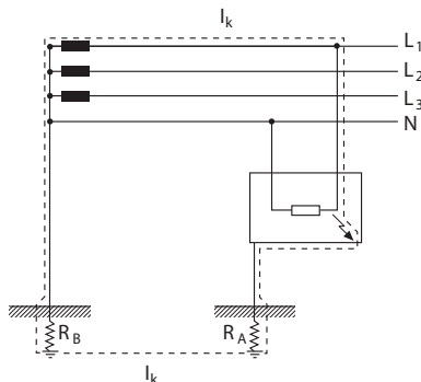
Рисунок 1: Замыкание на землю в системе ТТ
