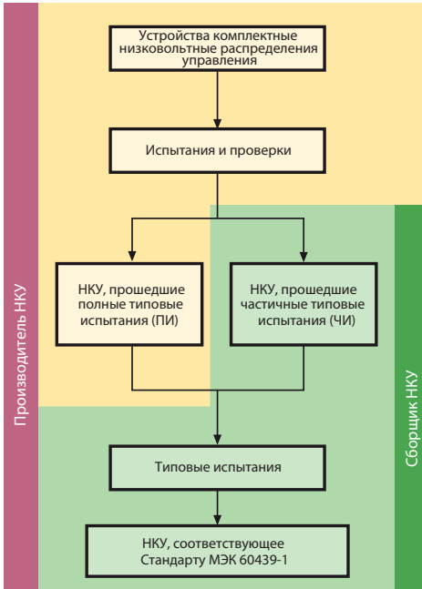
Стандарт МЭК 60439-1
