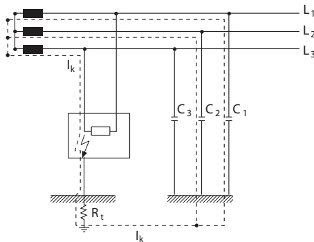
Рисунок 3: Замыкание на землю в системах IT
