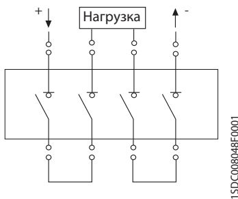
F) 2+2 последовательно соединенных полюса (1000 В пост. тока)
