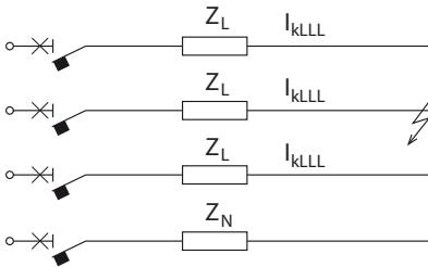
Трехфазное замыкание
