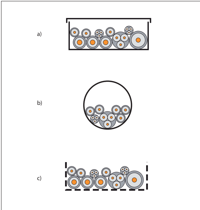
Кабели в пучке: а) в коробе; б) в канале; в) на перфорированном лотке
