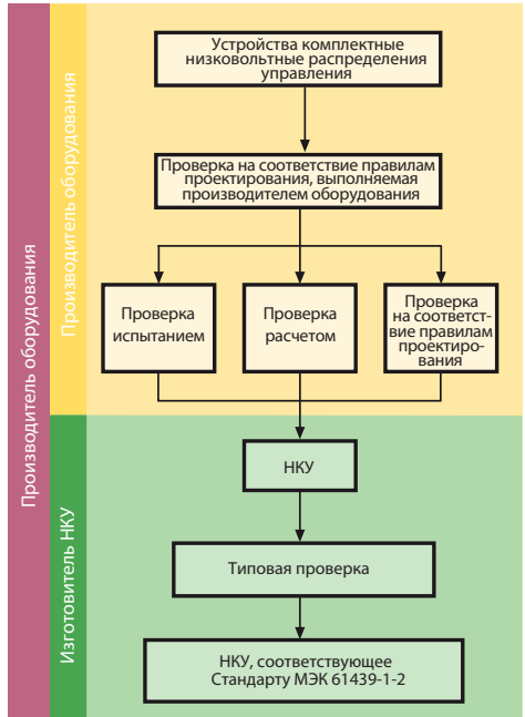
Стандарт МЭК 61439-1-2
