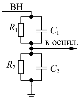
Рис. 3.13. Схема замещения смешанного делителя напряжения
