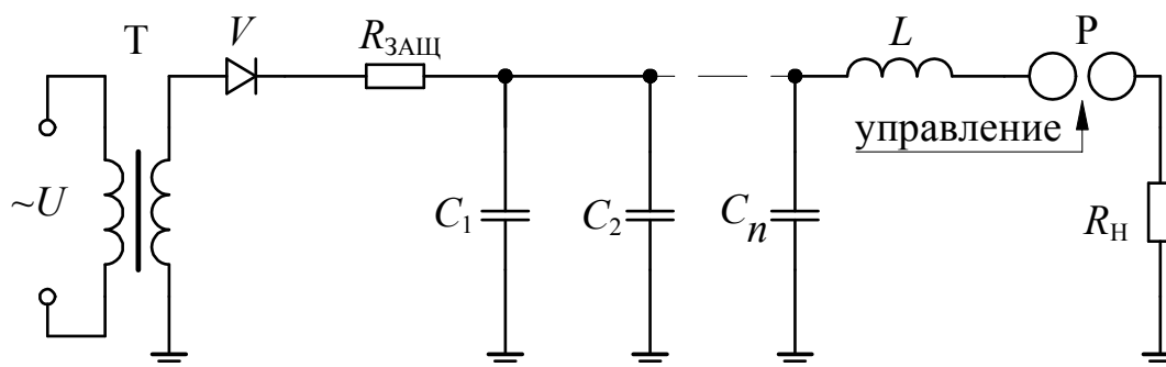
Рис. 3.8. Электрическая схема ГИТ: V – высоковольтный выпрямитель; R_{ЗАЩ} – сопротивление для ограничения зарядного тока; C_1 - C_n – батарея конденсаторов; P – разрядник управляемый; R_n – нагрузка; L – индуктивность разрядного контура
