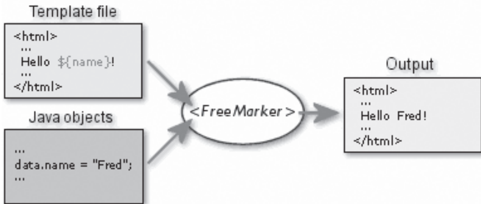
Рис. 2.4. Структура работы библиотеки FreeMarker
