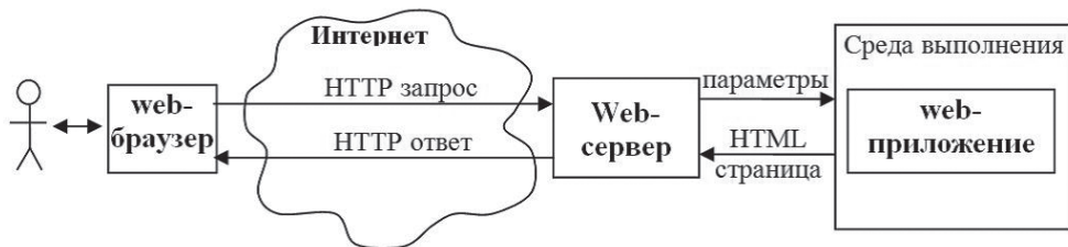
Рис. 1.2. Общая схема взаимодействия пользователя с Web-приложением
