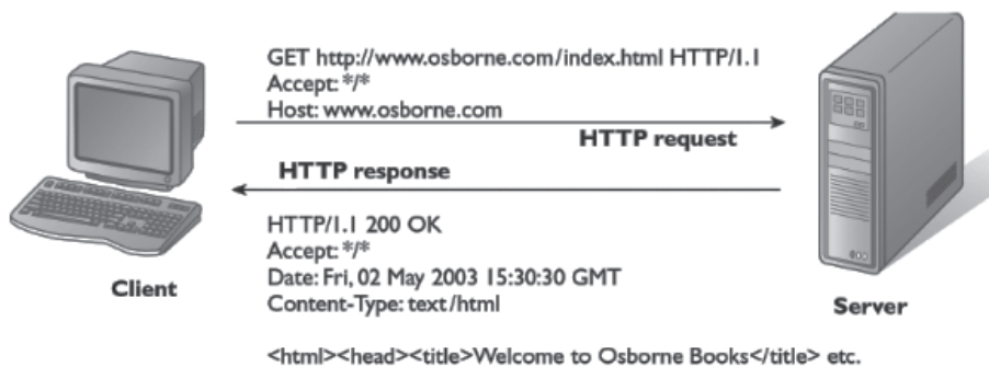
Рис. 1.1. Пример общения клиента и сервера по HTTP-протоколу
