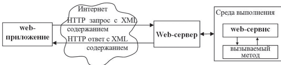
Рис. 1.3 Общая схема взаимодействия пользователя с web-сервисом
