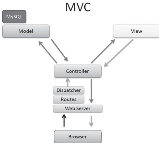
Рис. 1.5. Структура MVC-модели
