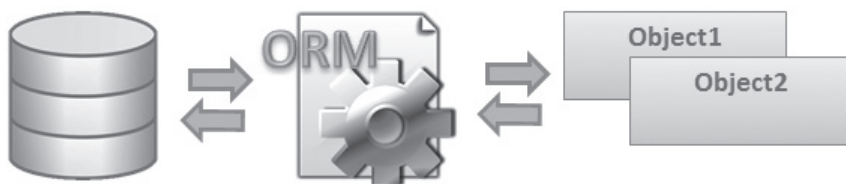
Рис. 1.6. Структура ORM-технологии
