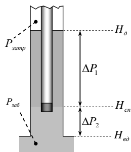
Рис. 1. – Определение забойного давления механизированной скважины
