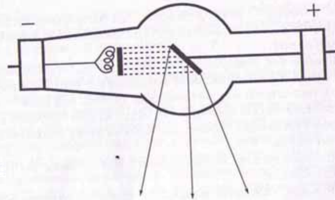
Рис. 1.4. Схема образования рентгеновских лучей в рентгеновской трубке
